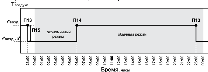
Рис.6 График температуры воздуха в помещении для Режим 2.
