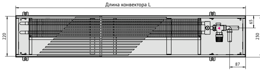
Вид сверху конвектора Ntherm Maxi 230 с роликовой решеткой, с U-образным бортом.
