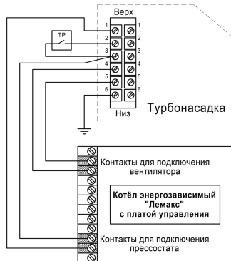
Схема подключения турбонасадке "Лемакс" к котлу с платой управления
