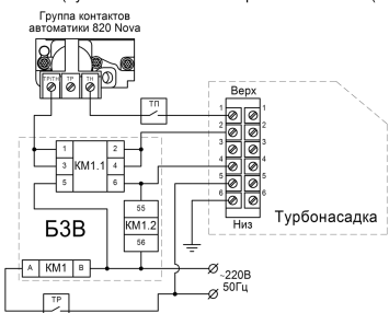
Схема подключения турбонасадке "Лемакс" к котлу с автоматикой безопасности SIT 820 Nova и блоком задержки времени (пускатель ПМЛ-1100 и приставка ПВЛ-22(21))
