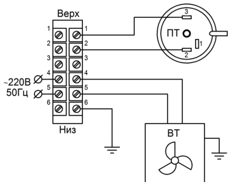
Схема турбонасадке "Лемакс" для энергозависимого котла
