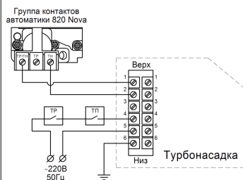
Схема подключения турбонасадке "Лемакс" к котлу с автоматикой безопасности SIT 820 Nova
