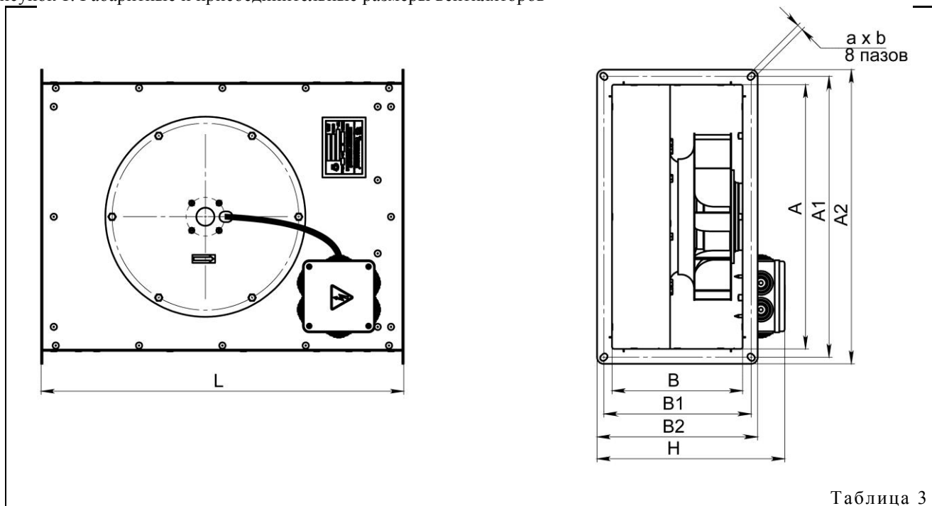
Рисунок 1. Габаритные и присоединительные размеры вентиляторов
