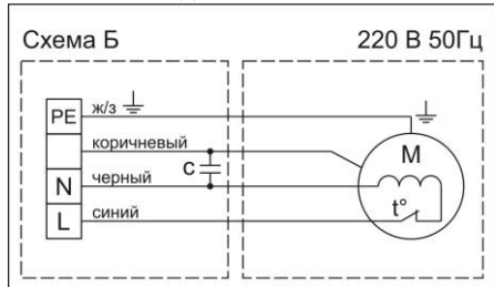
Схема Б. Подключение к сети 220
