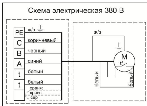
Подключение к сети 380 В;
