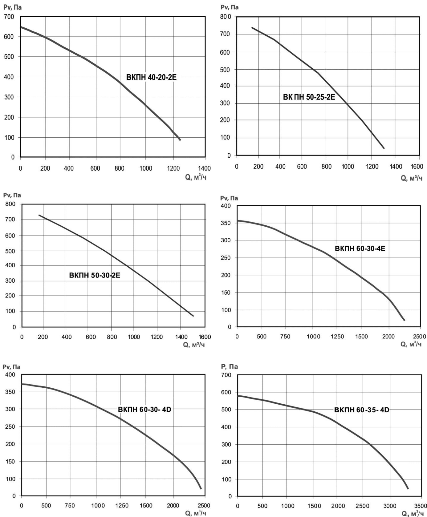
Рисунок 3. Аэродинамические характеристики вентиляторов канальных прямоугольных с вперед загнутыми лопатками (статическое давление от производительности)
