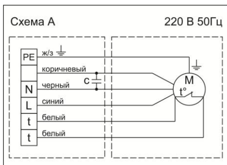
Схема А. Подключение к сети 220 В
