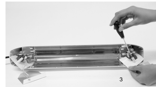
3. ОТКРУТИТЕ ВИНТЫ, НАХОДЯЩИЕСЯ В ЗАЖИМАХ БОКОВЫХ ЧАСТЕЙ КОРПУСА И ЗАКРЕПЛЯЮЩИЕ ДВА ПРОВОДА ЛАМПЫ
