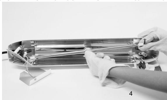
4. ИЗВЛЕКИТЕ ЛАМПУ, ОТСОЕДИНИВ ЕЕ ОТ ПРУЖИН. ВСТАВЬТЕ НОВУЮ ЛАМПУ В ПРУЖИНЫ ТАК, ЧТОБЫ ПРЕДВАРИТЕЛЬНО УКОРОЧЕННЫЕ ПРОВОДА ЛАМПЫ БЫЛИ ВТАВЛЕНЫ В ЗАЖИМЫ. СОБЕРИТЕ ЗАНОВО ОБОРУДОВАНИЕ, ПОВТОРИВ ВЫШЕ ПЕРЕЧИСЛЕННЫЕ ОПЕРАЦИИ В ОБРАТНОМ ПОРЯДКЕ ОТ ОПИСАННОГО.
