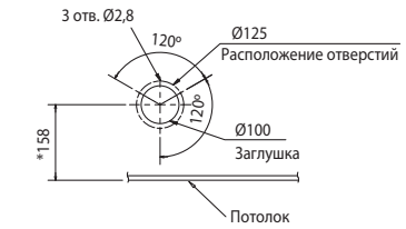
Подключение приточного воздуховода
