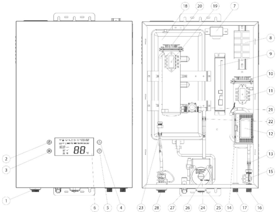
Рис. 1. Конструкция изделия
