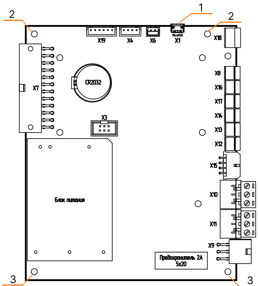
Рис.13 Плата контроллера
