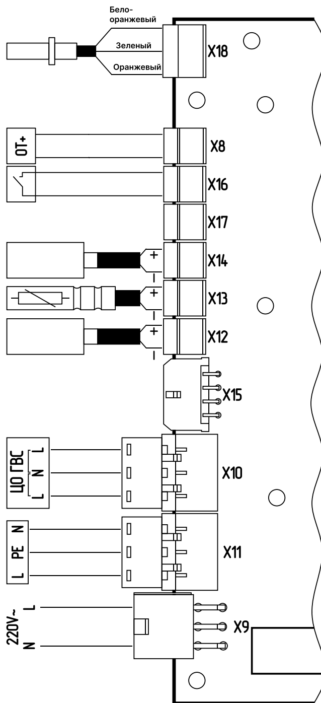
Рис.4 Схема подключения датчиков «ZOTA X-Line100E».
