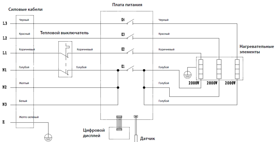
Рисунок 3. Электрическая схема подключения
