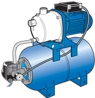
Модель Uni-Jet ... S корпус насоса - нерж.сталь
