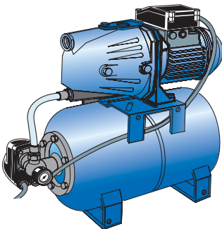
Модель Uni-Jet ... G корпус насоса - окрашенный чугун
